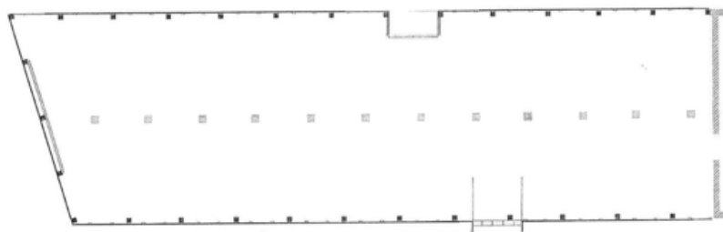
Plantegning 1:200
