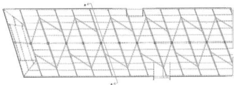
Hovedkonstruksjon tak og sprengverk, med åser lagt oppå sprengverket målestokk 1:200
