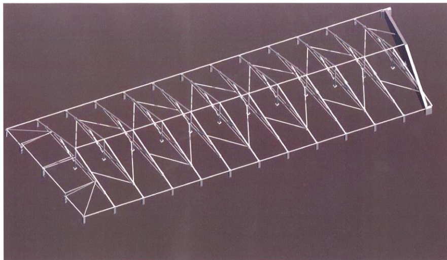
Aksionometrisk oppbygging
