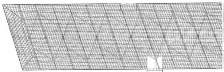
Hovedkonstruksjon tak og sprengverk, med strøbord lagt oppå åsene målestokk 1:200
